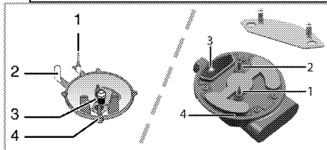
1 Gasdurchfluss-Einstellschraube
