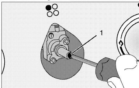
1 Stelschroef gasdebit
