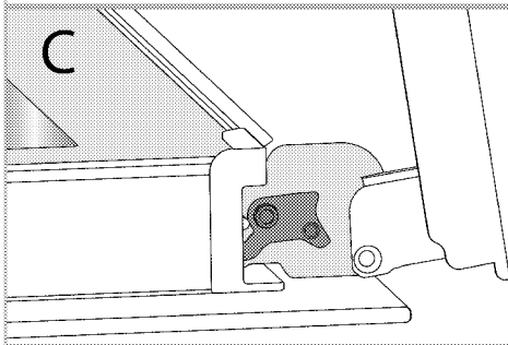
Schamiervergrendeling - open positie 3.Laat de ovendeur half open staan.
