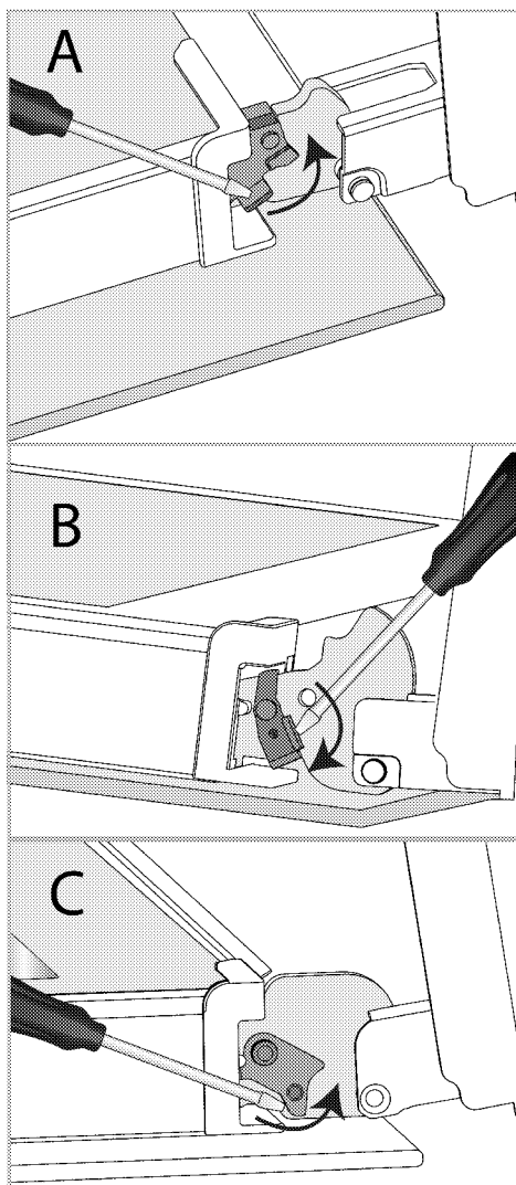
Scharniergevendeling - gesloten positie
