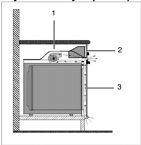
1 Cooling fan
