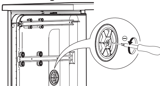
Abbildung 2: Mechanische Einstellgrafik
