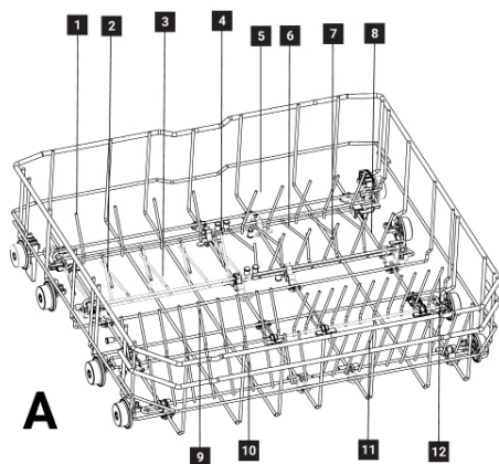
Abbildung 4: Anzahl der klappbaren Drähte im unteren Korb
