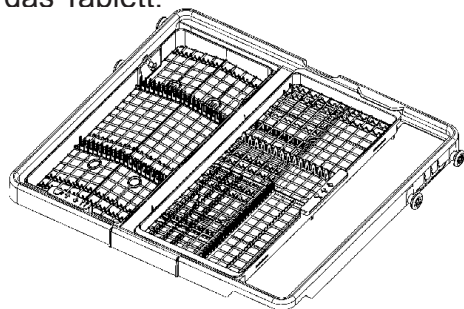
Abbildung 10: Decken-Besteckkorb Das rechte Tablett lässt sich seitlich frei verschieben. Durch das Verschieben nach links entsteht darunter zusätzlicher Platz für größere Gläser im Oberkorb. Ein weicher Spike hält das Tablett.
