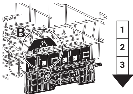
Abbildung 7: Verringern der Stufen des oberen Korbs.
