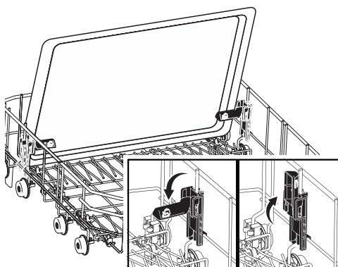
Abbildung 11: Backblech-Waschhalter
