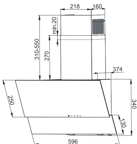
Abb. 2 Dimensionszeichnung
