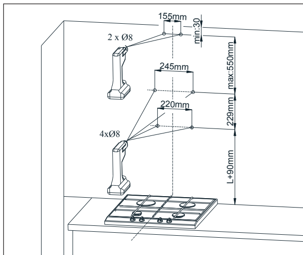
Abb. 5 Spreizschrauben montieren
