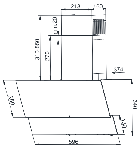
Afb. 2 Afmetingenschema
