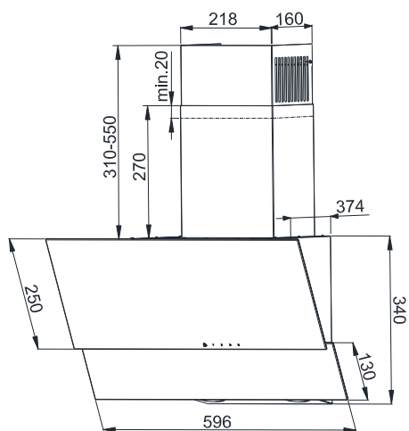
Obr.2 Rozmer kreslenia
