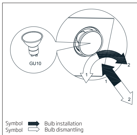
Abb. 11 Leuchtmittel auswechseln
