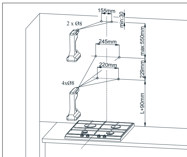
Afb. 5 Montage van de verlengingsbouten
