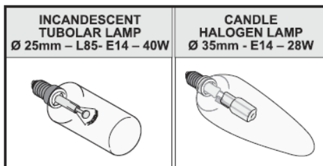
Cevasta žarnica
