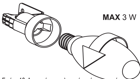
Εικόνα 12: Αντικατάσταση λαμπτήρα τύπου κεριού
