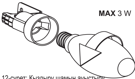
12-сурет: Қыздыру шамын ауыстыру
