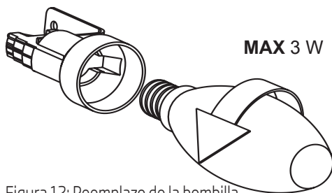
Figura 12: Reemplazo de la bombilla
