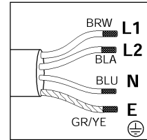
2 N AC 220-240 V / 380-415 V
