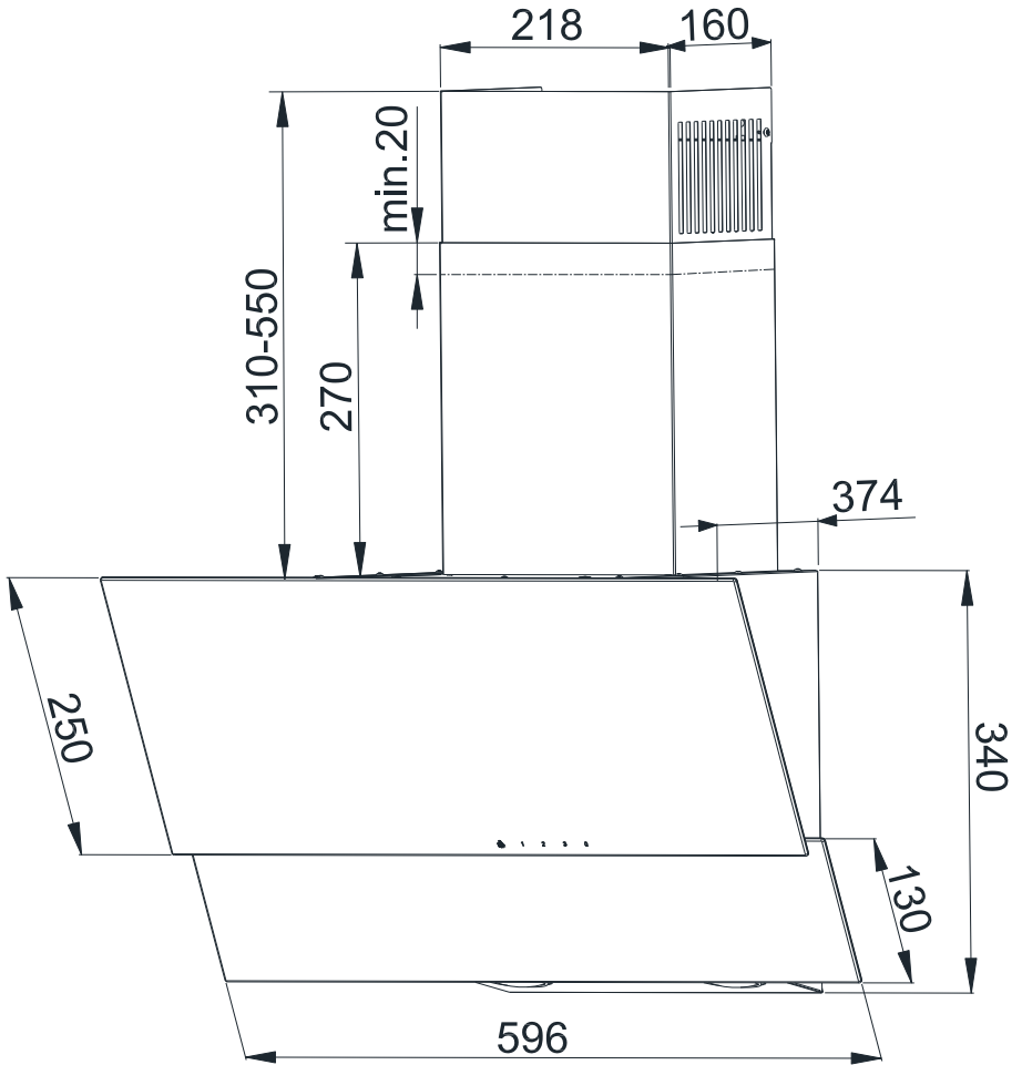
Abb. 2 Dimensionszeichnung
