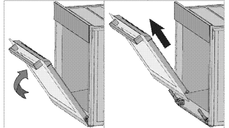
Scharnivergrendeling - open positie 3. Laat de ovendeur half open staan.
